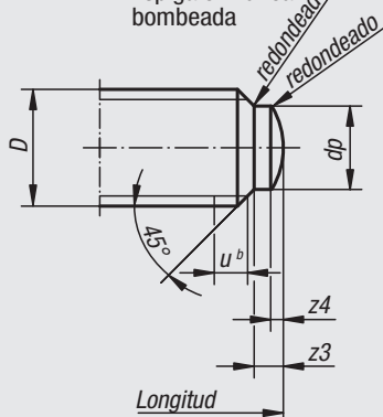
Ak Espiga cilíndrica bombeada
