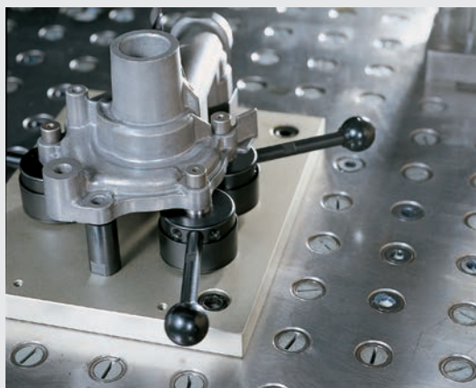
Ejemplo de aplicación de sujeción por tracción
