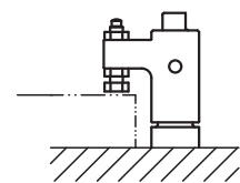
3. Fijar el tornillo de sujeción mediante las tuercas hexagonales.
