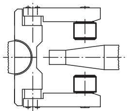
Posición del punto cero del soporte con bola oscilante
