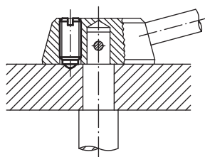
Bloqueo de la palanca de mando
