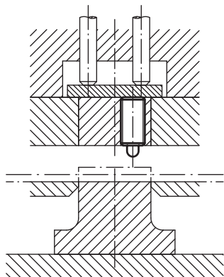
Pasador de presión en sección completa
