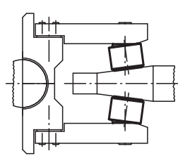
El soporte con bola oscilante se adapta al contorno de la pieza de trabajo
