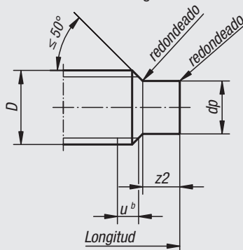
Ak Espiga cilíndrica bombeada
