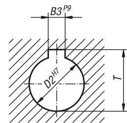
DIN 6885-1
