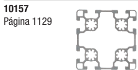
Perfiles de aluminio 90x90 ligeros Tipo B
