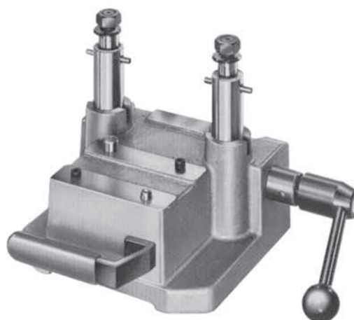
Tamaño 3 S: 125 x 100 x 72 mm
