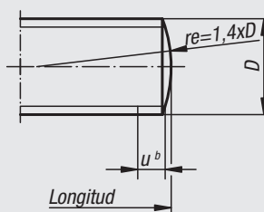
LD Pivote largo
