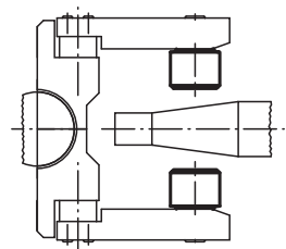
Retorno automático del soporte con bola oscilante
