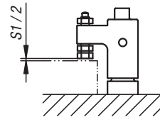
2. Girar el brazo de sujeción manualmente a la posición "cerrar". Ajustar la distancia entre el tornillo de sujeción y la pieza de trabajo a la mitad del recorrido de sujeción (S1).
