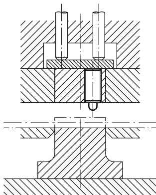
Pasador de presión en sección completa
