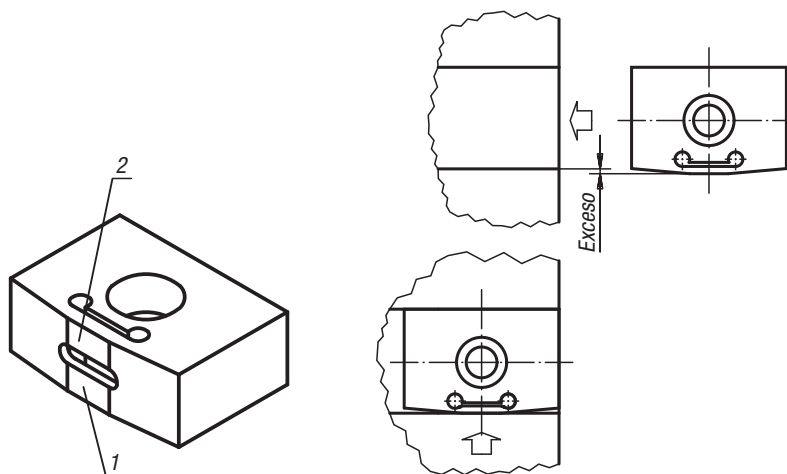
Alojamiento sin juego mediante deformación elástica
