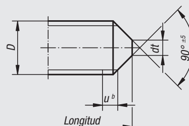
TC Punta aplanada
