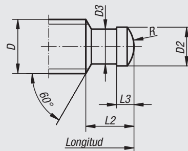
Pivote opresor según DIN 6332
