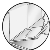
Conexión elástica e impermeabilización
