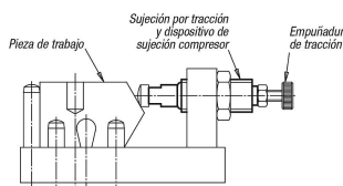
Sujeción por tracción y dispositivo de sujeción compresor
